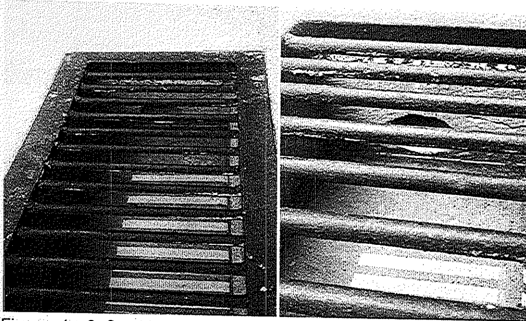
Figuras 1 y 2: Sumideros inundados por mala colocación del desagüe
