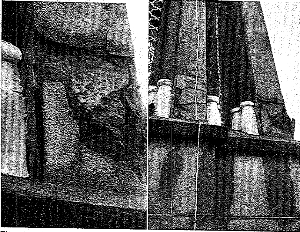
Figuras 5 y 6: Forro en granito de mala calidad.
